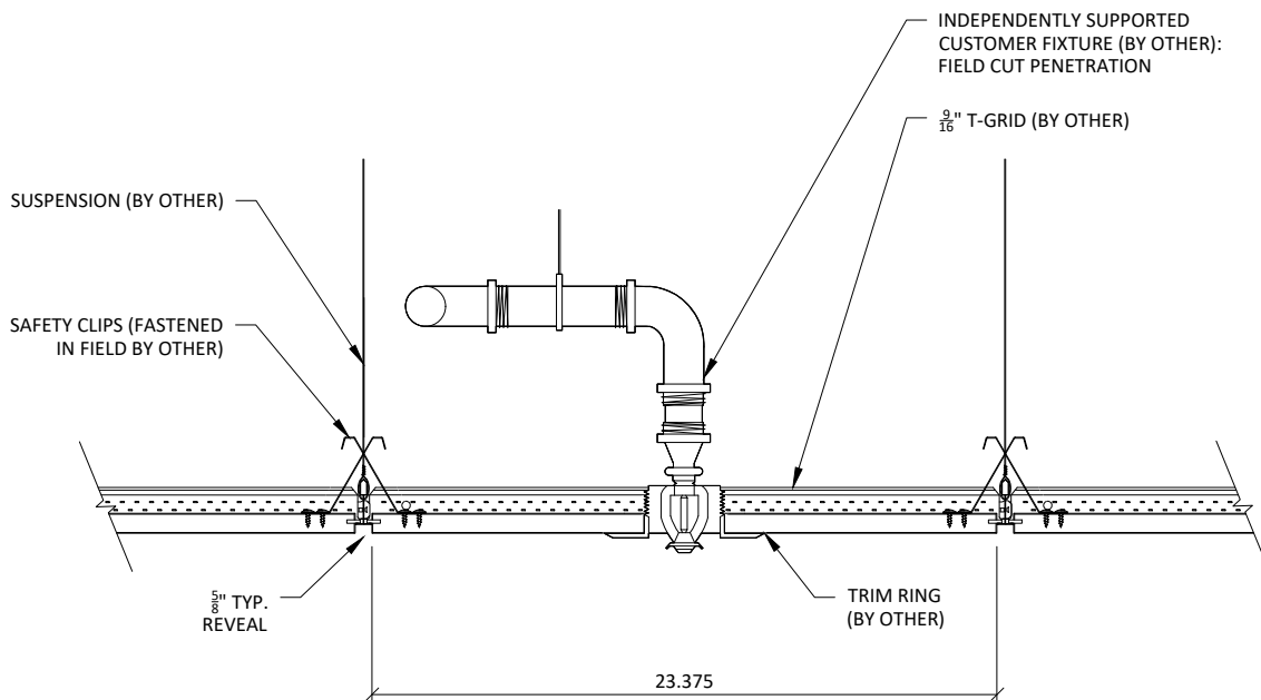
2 SPRINKLER SECTION SCALE: 1 1/2" = 1' 0"
