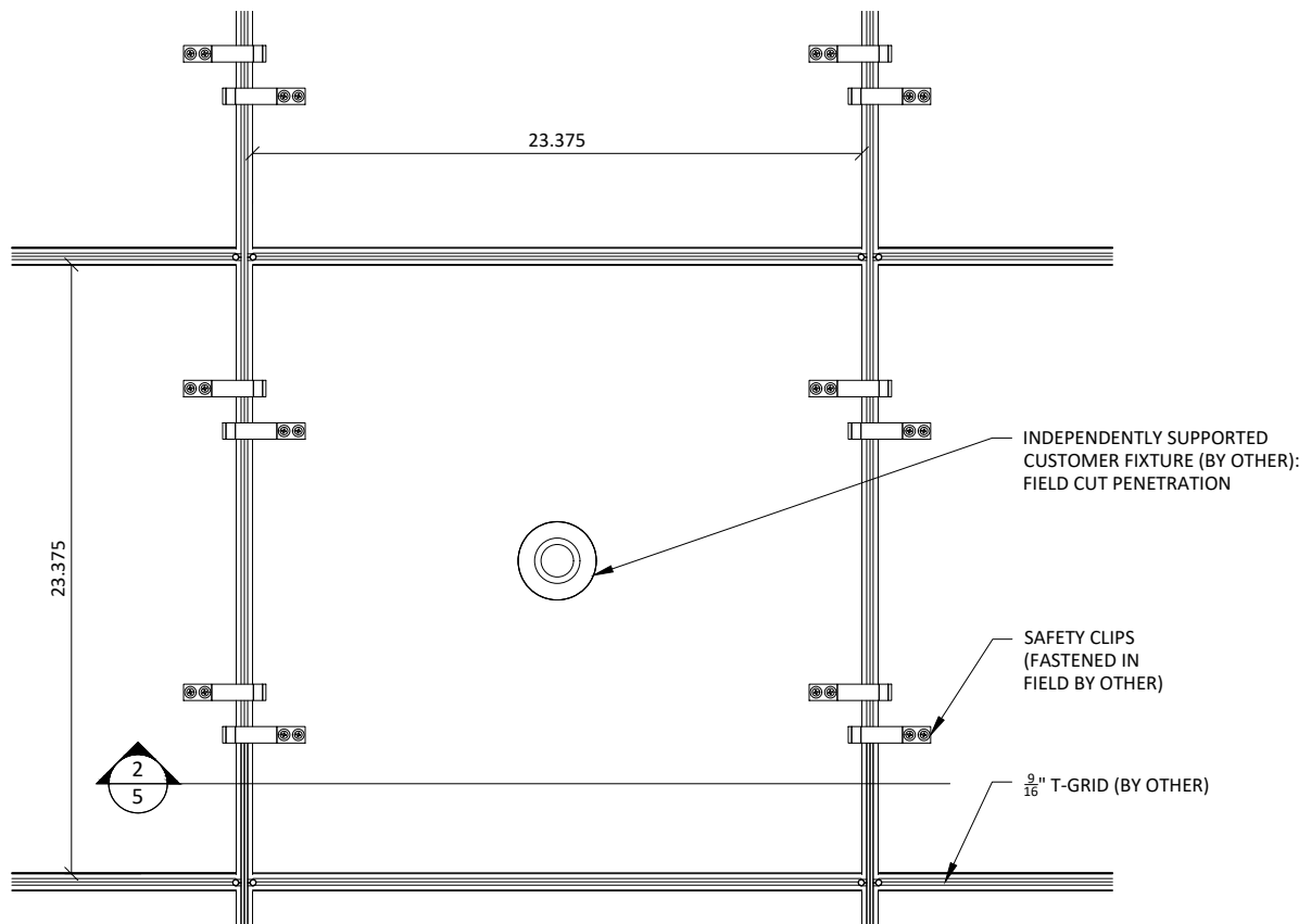
1 SPRINKLER PLAN SCALE: 1 1/2" = 1' 0"
