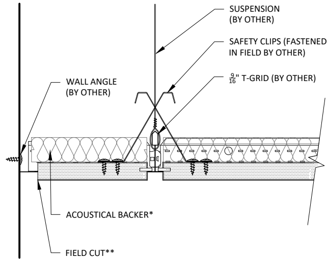
1 4 EDGE DETAIL SCALE: 3" = 1' 0"
