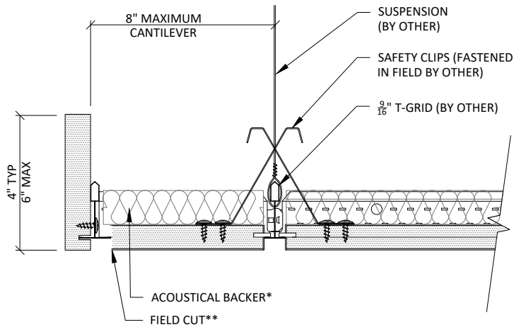
2 4 TRIM DETAIL SCALE: 3" = 1' 0"
